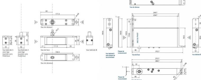
Pivot supérieur
