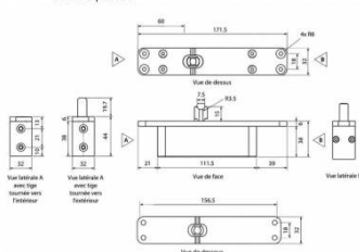
Pivot supérieur
