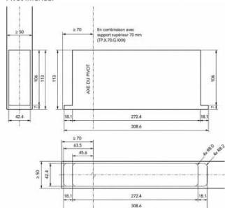
Pivot inférieur
